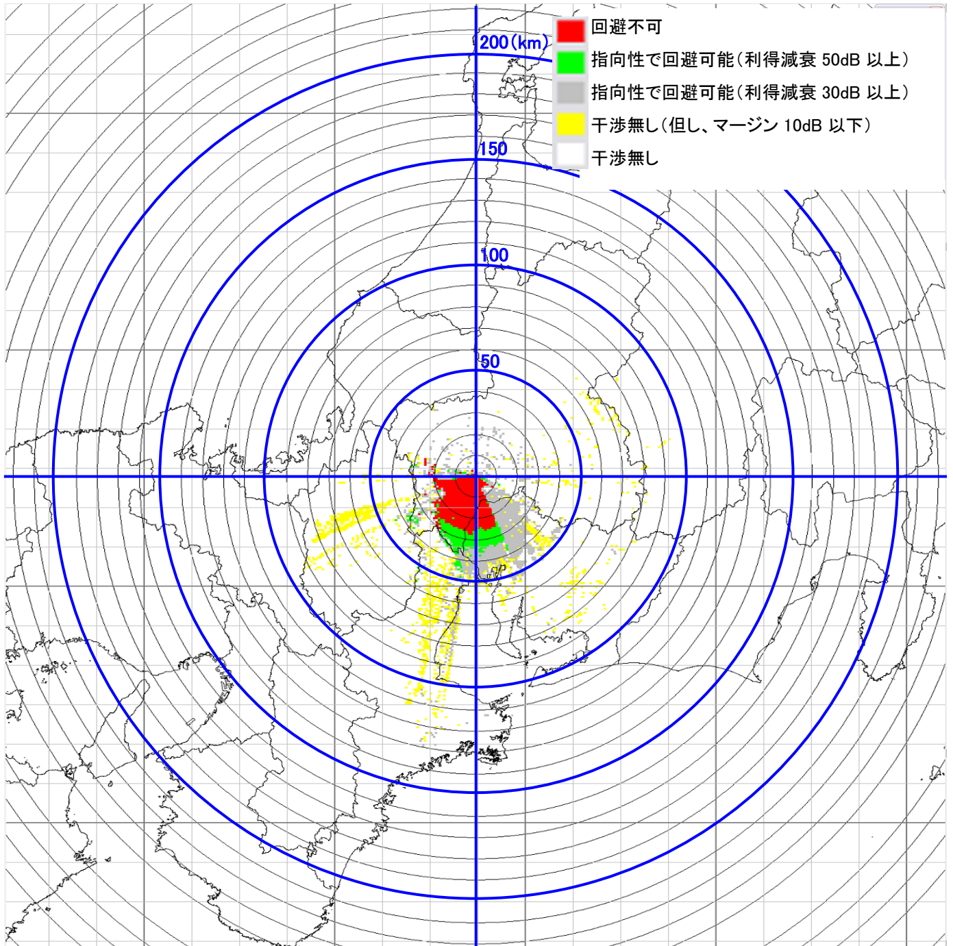
13-① 岐阜大岐阜 電界強度マップ・・・φ60cm パラボラアンテナ送信機
